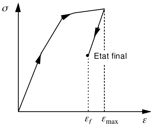
Elasto-plasticité
