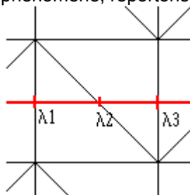
Figure 7 - Les 3 nœuds se voient imposer la relation linéaire \lambda_1 - 2\lambda_2 + \lambda_3 = 0 par l'algorithme de stabilisation de la LBB.
