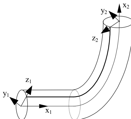
Figure 3.2.2-b : Représentation de la génératrice de référence.
