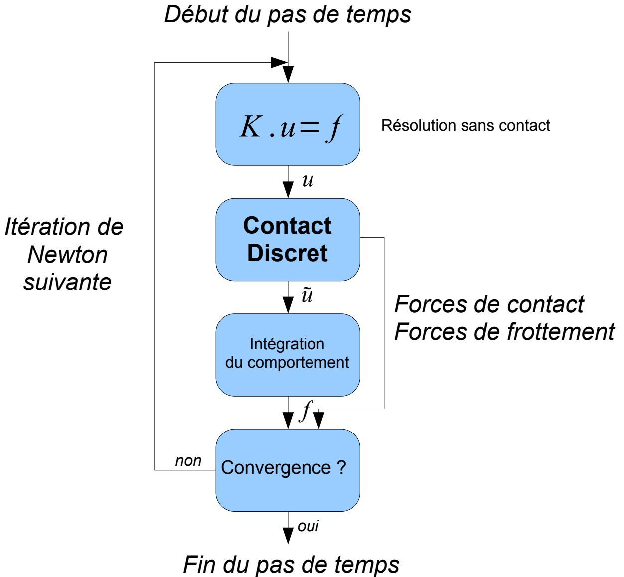
Figure 3.1.2-1: Algorithme général d'un pas de temps en formulation discrète (petits glissements)
