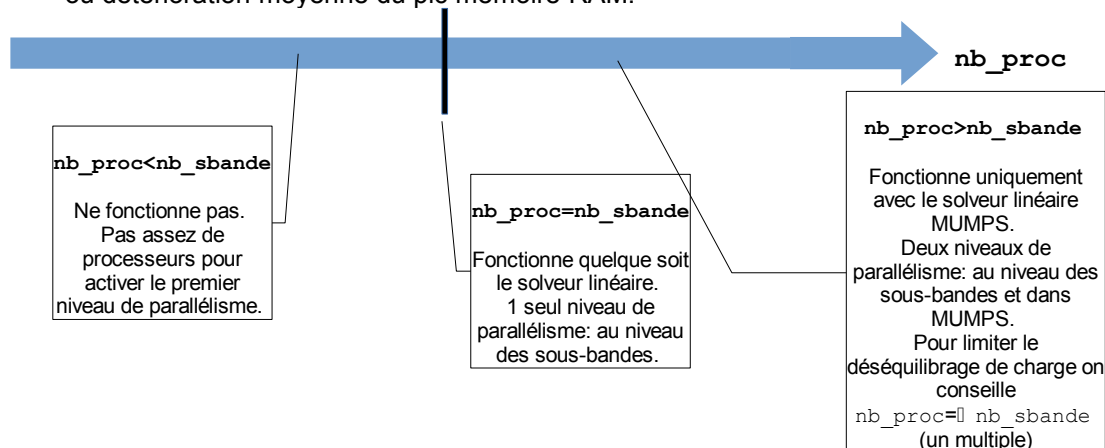
Image 3.12-2 - Périmètre d'utilisation avec NIVEAU_PARALLELISME='COMPLET' .
