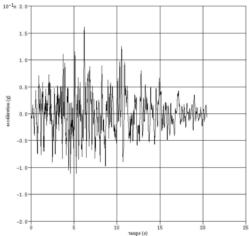
Figure 1.3-c : Accélérogramme acc3.c2
