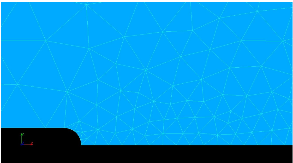
Figure 4.2 : Zoom sur l'entaille du maillage initial.
