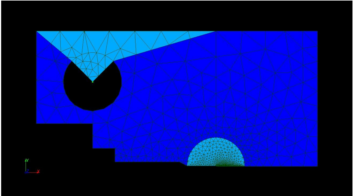
Figure 4.1 : Vue d'ensemble du maillage initial.
