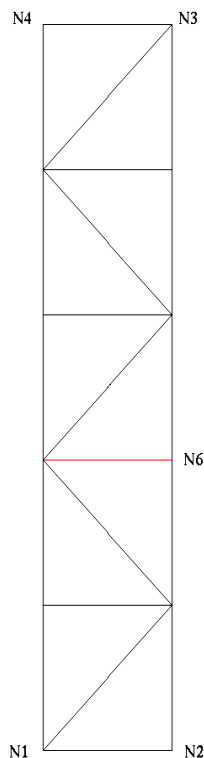
Figure 12.2-a: Maillage de la modélisation J
