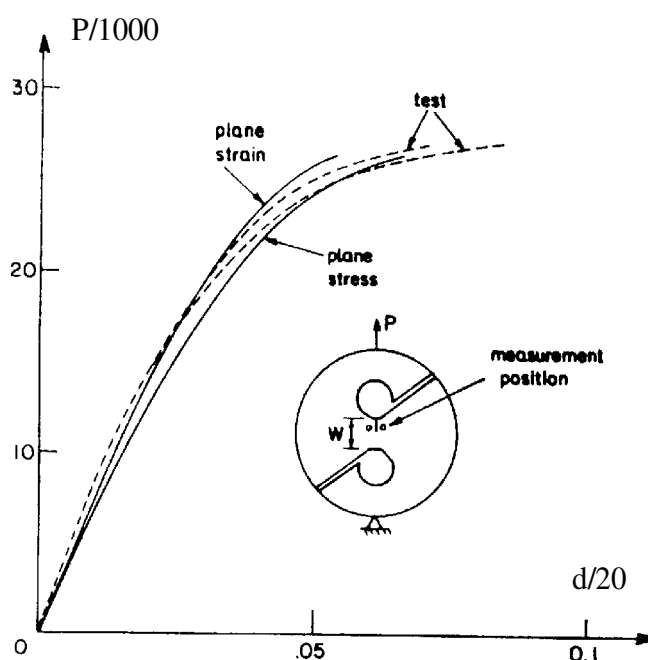
Courbe de réponse charge/déplacement
