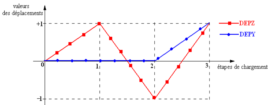
Figure 1.3-1: Variations des chargements en déplacements imposés
