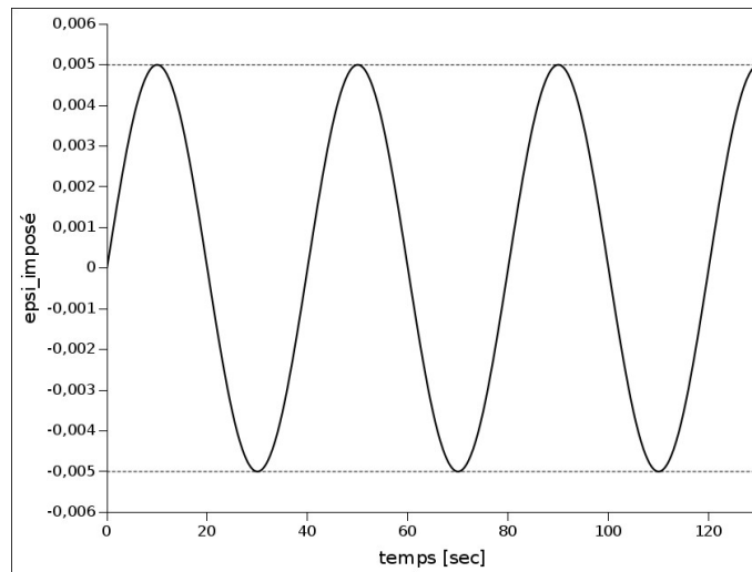
Figure 1.3.9-1: Trajet de chargement 9
