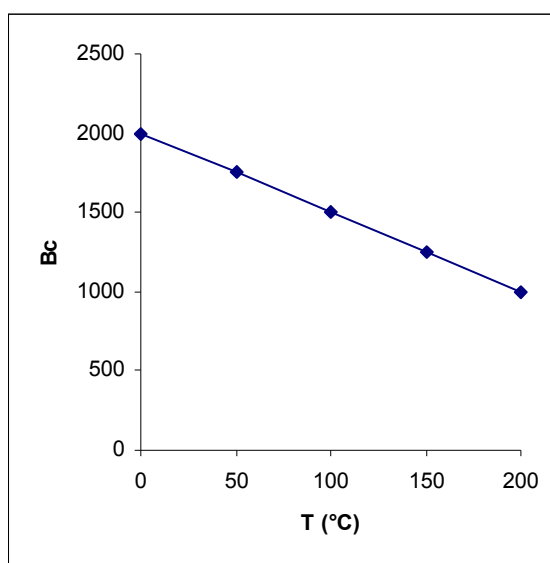
Figure 1.2-b : Evolution de B_C avec la température
