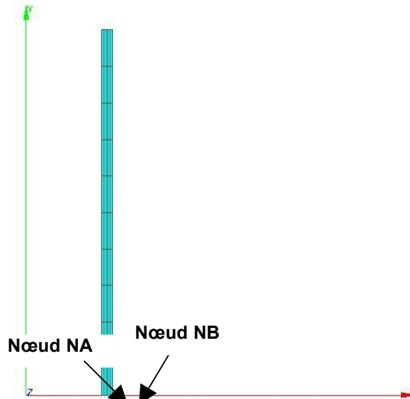
Figure 3.1-a : Géométrie et maillage de la modélisation
