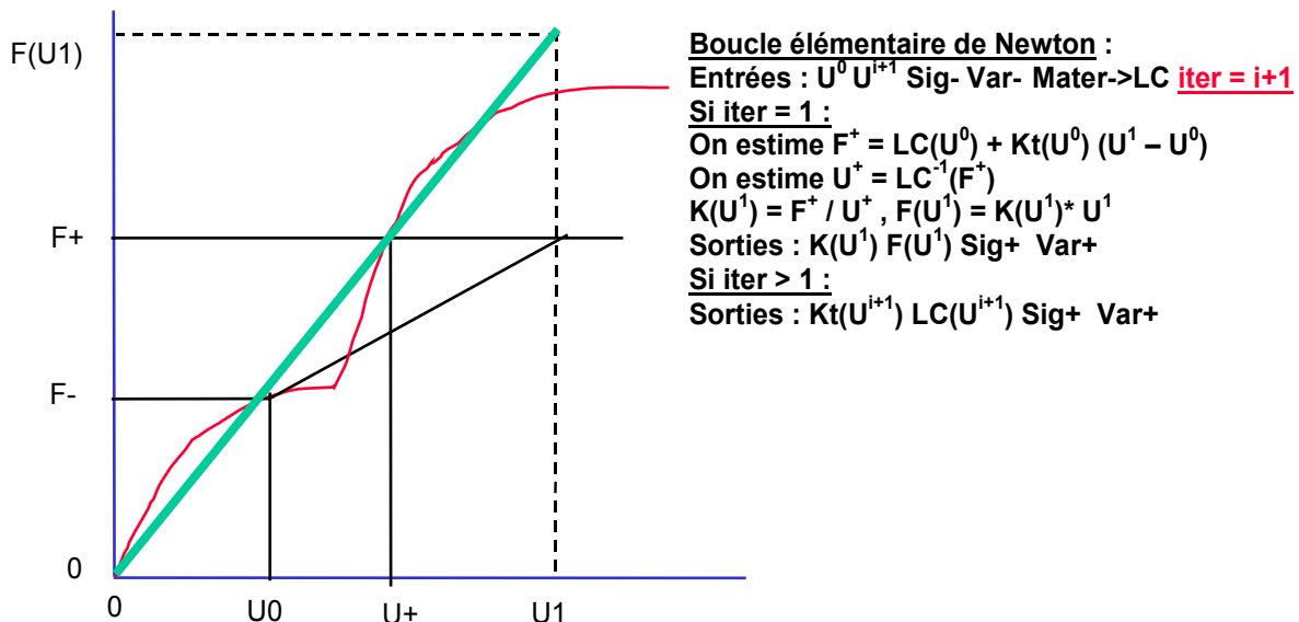
Figure 4.3-a : méthode de sécante dirigée
