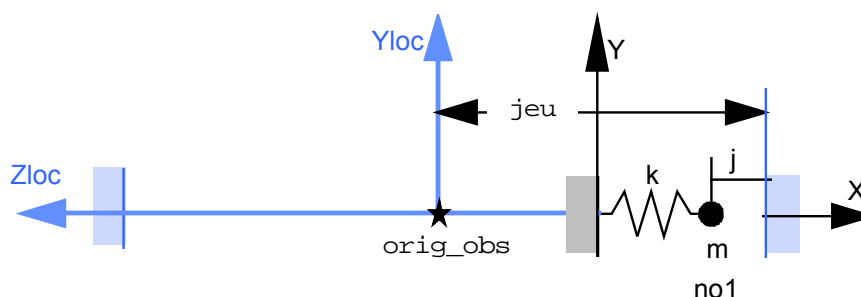
Figure 3.6.1.6-a : Système masse-ressort impactant une paroi fixe
