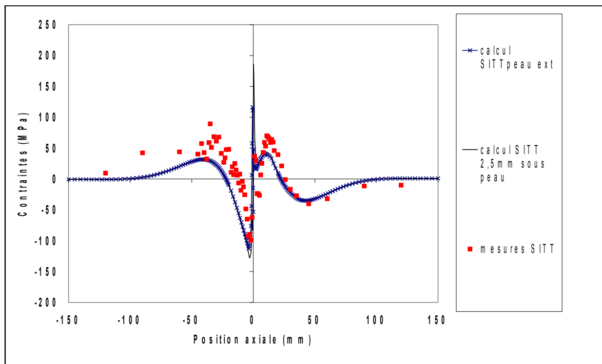
Figure 4.2 : Profil des contraintes circonférentielles calculées et mesurées en peau externe
