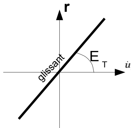
Figure 4.3.3.2-a : régularisation de la condition d'adhérence – Modèle de Tresca.
