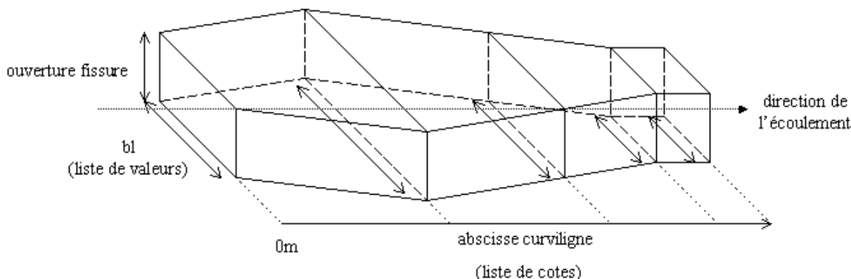
Figure 3.15.4-1: Représentation de la fissure
