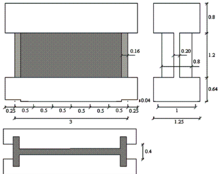
Figure 1.1-a: Géométrie de la maquette T5
