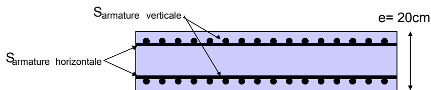
Coupe dans le plan horizontal du mur central Figure 1.1-b: Illustration du ferrailage
