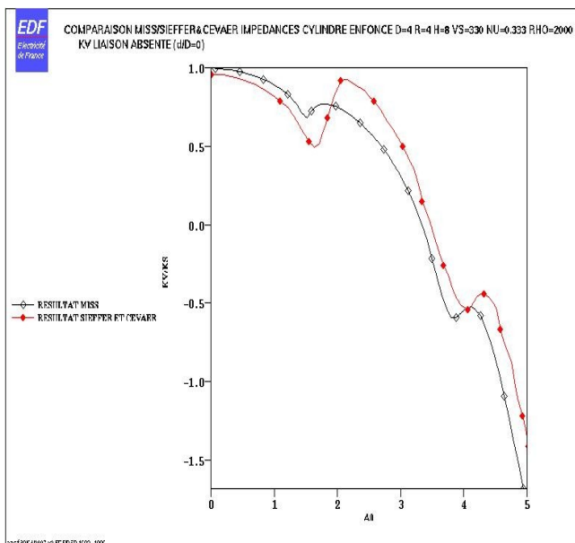
Figure 3.1-b : Évolutions des impédances de translation verticale
