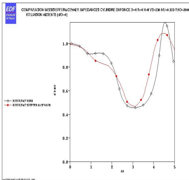
Figure 3.1-c : Évolutions des impédances de balancement
