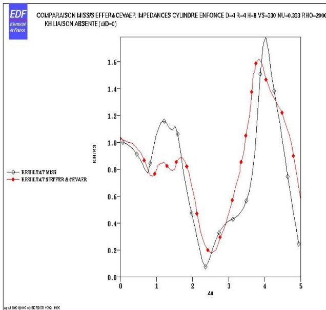
Figure 3.1-a : Évolutions des impédances de translation horizontale
