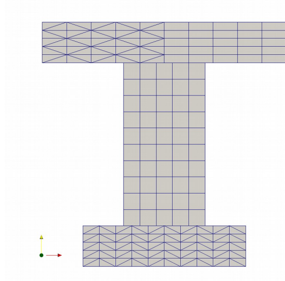
Figure 4-1: Section de la poutre pour SSL111b
