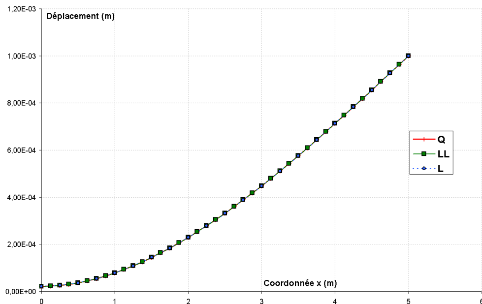
Illustration 1: Déplacement le long de la poutre
