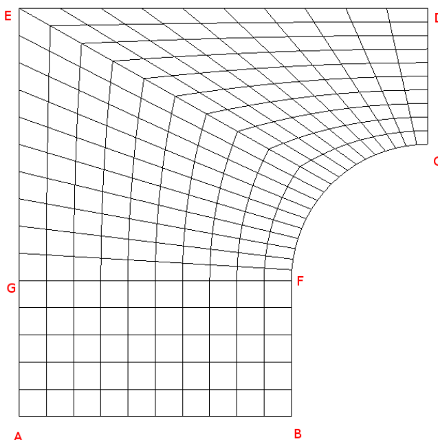
Figure 3.1-a : Maillage.
