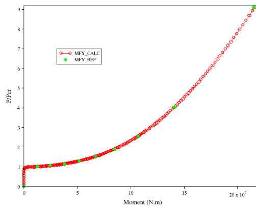
P/Pcr en fonction du moment MFY
