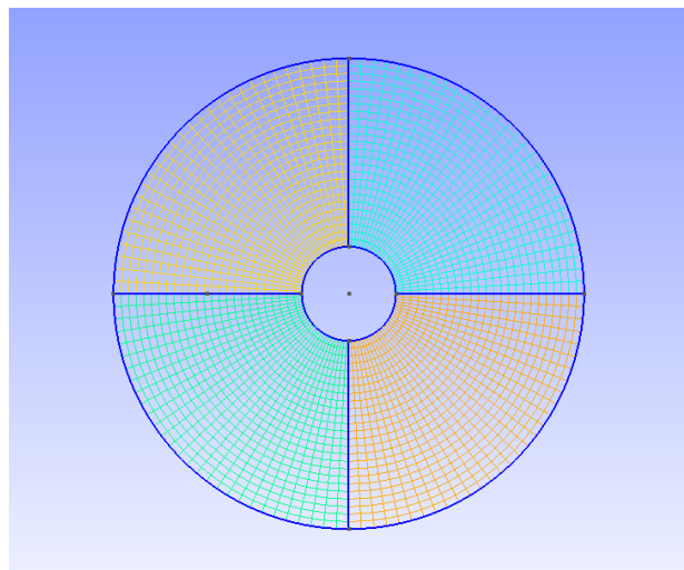
Figure 5.2-a: Le maillage de la modélisation C
