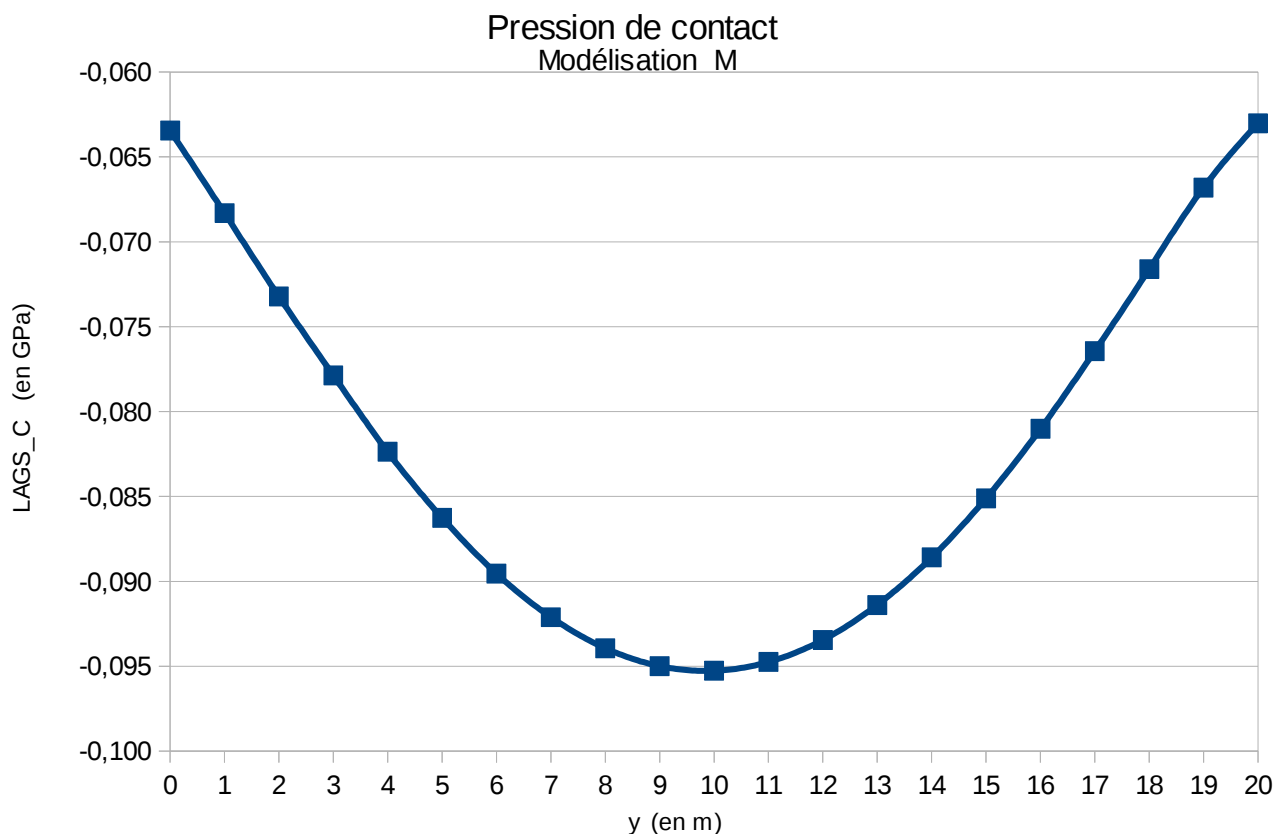
Figure 17.4-1: Evolution de la pression de contact suivant l'axe Oy.
