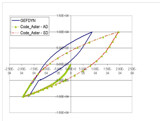
Figure 4-a : Contrainte déviatoire en fonction de la distorsion : comparaison des solutions de Code_Aster et GEFDYN
