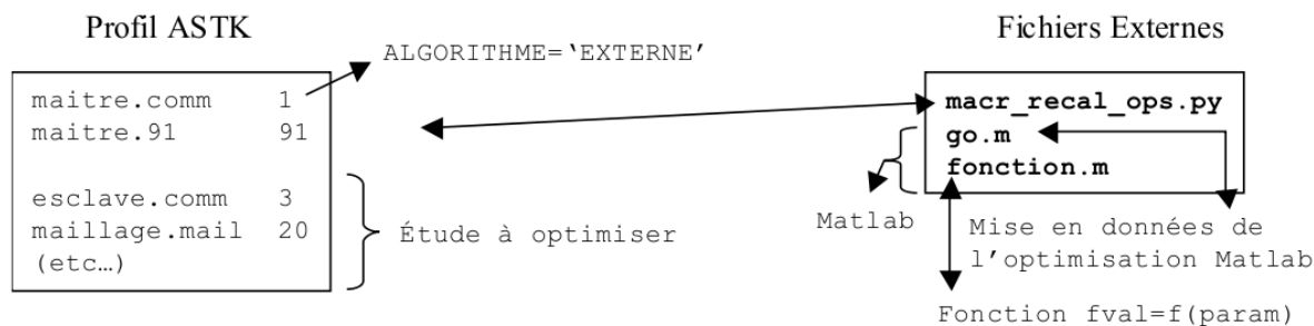
Figure 3.3-a : MACR_RECAL méthode EXTERNE
